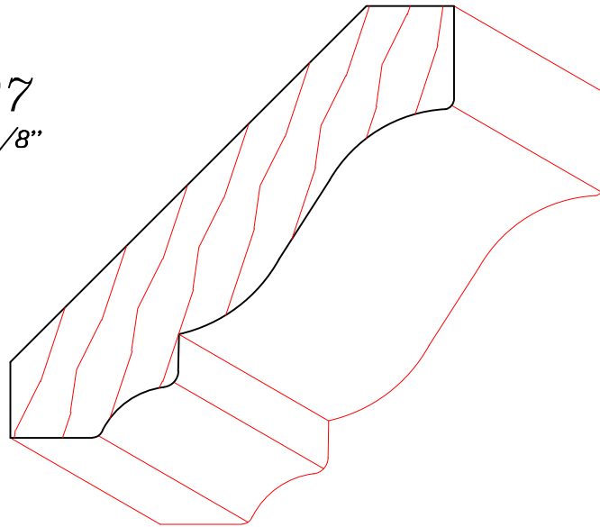
TM3088 3/4" X 3-9/16"
