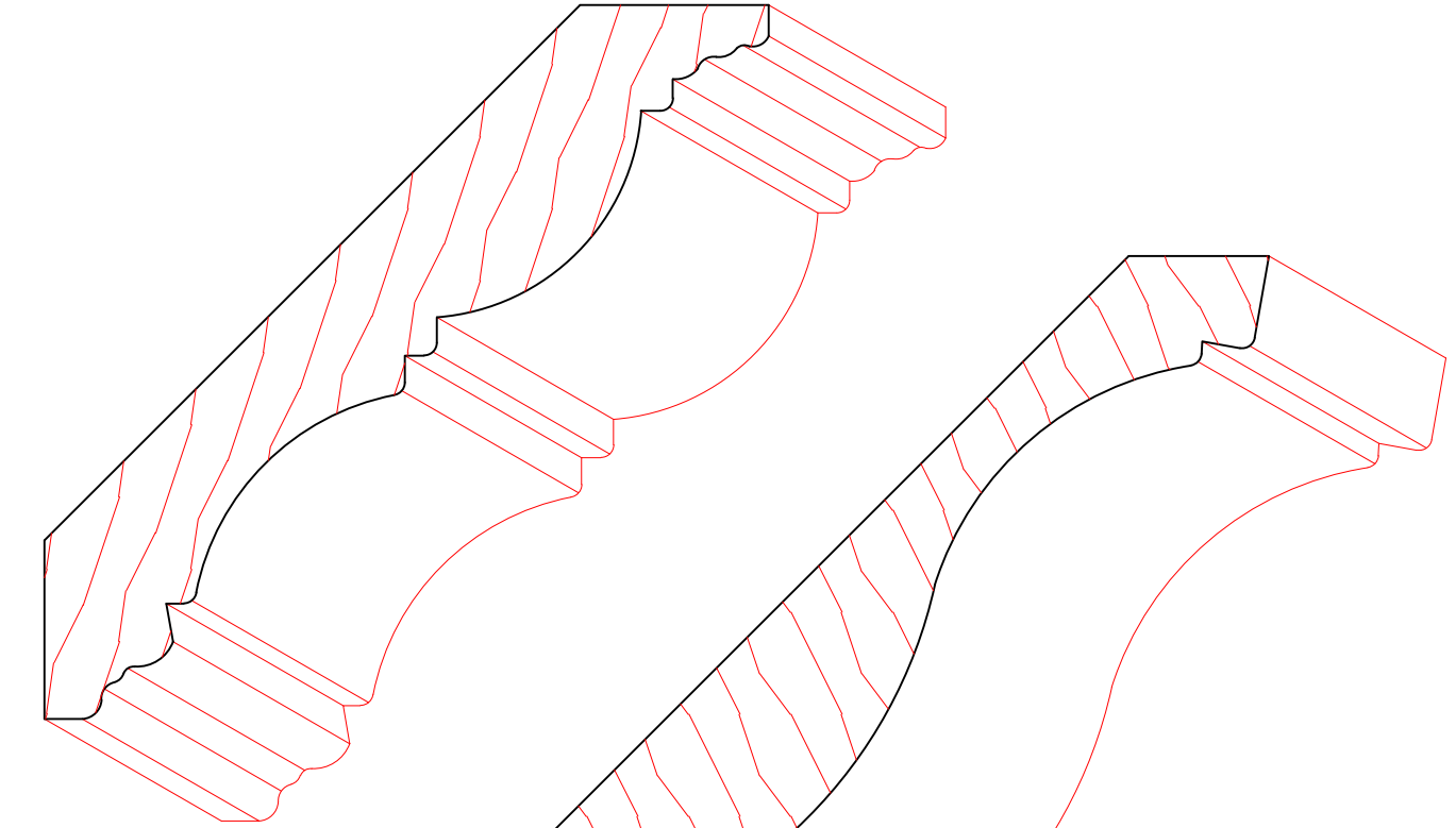
TM3057 13/16" X 5"
