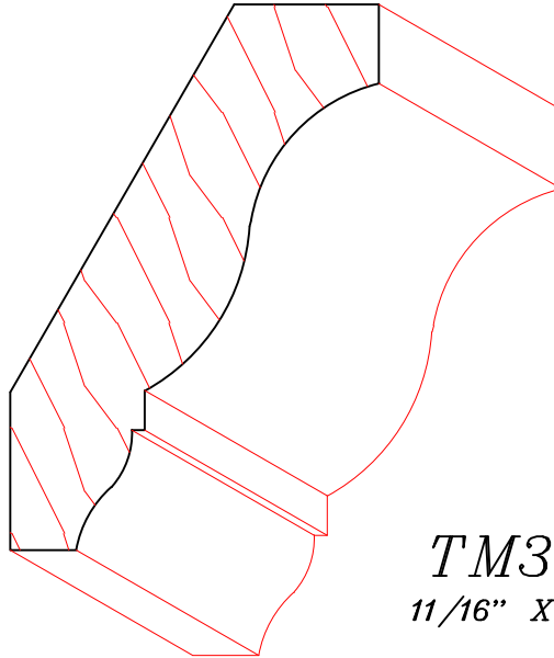
TM3015 3/4" X 5"
