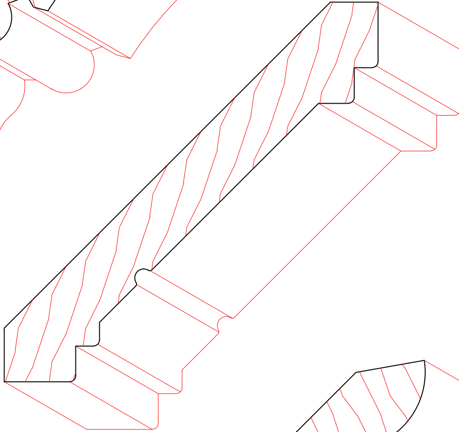
TM3085 3/4" X 5-9/16"
