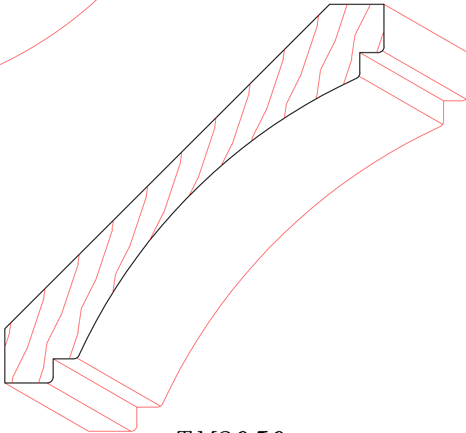
TM3050 3/4" X 5-9/16"
