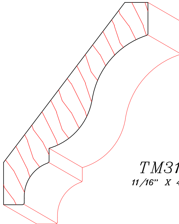
TM3136 9/16" X 2-15/16"
