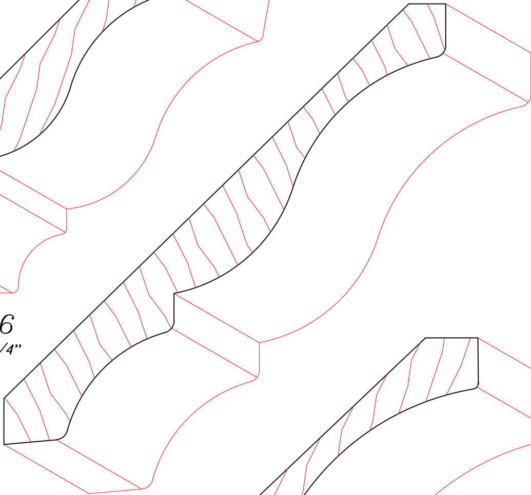
TM3067 3/4" X 6-5/16"
