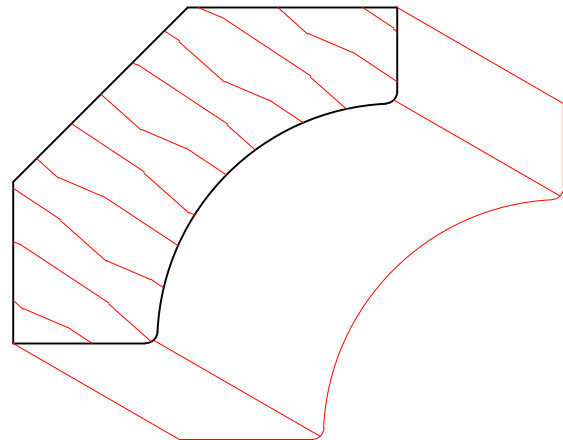
TM3103 1-1/16" X 2-11/16"
