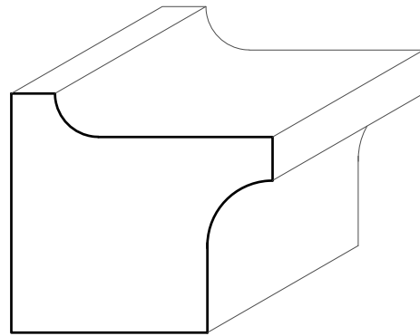
TM6059 1-1/2'' \times 1-3/8''
