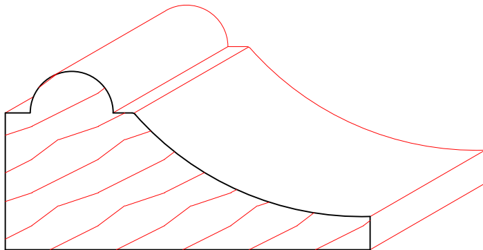
TM6034 1-3/8" X 2-3/4"
