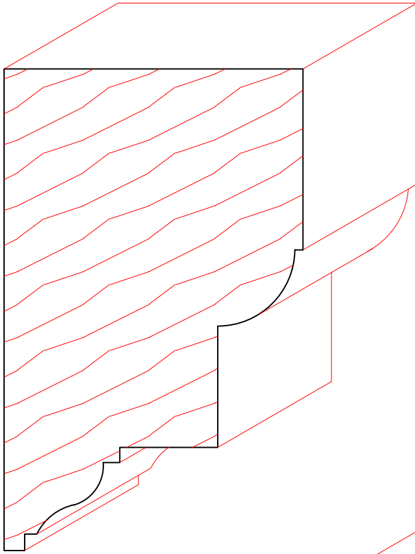
TM6054 2-1/4" x 3-11/16"
