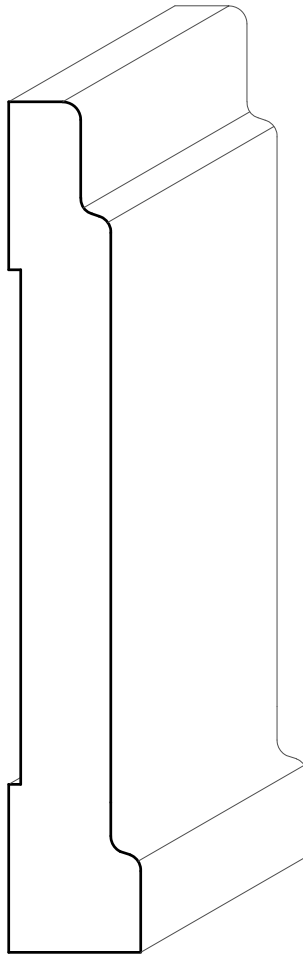
TM2093 11/16" X 4-1/2"
