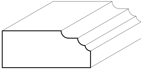
TM7161 5/8'' \times 1\text{--}1/2''
