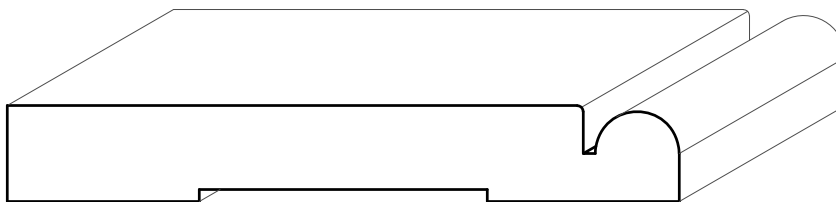
TM1087 1/2'' \times 3-1/2''
