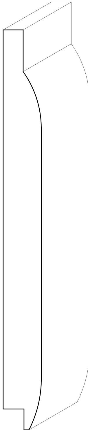
TM8099 11/16" X 7-3/16"
